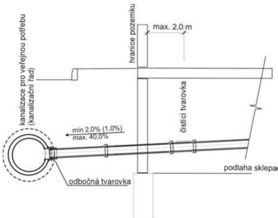
c) Schéma s čistící tvarovkou na kanalizační přípojce v půdorysu objektu nad podlahou
