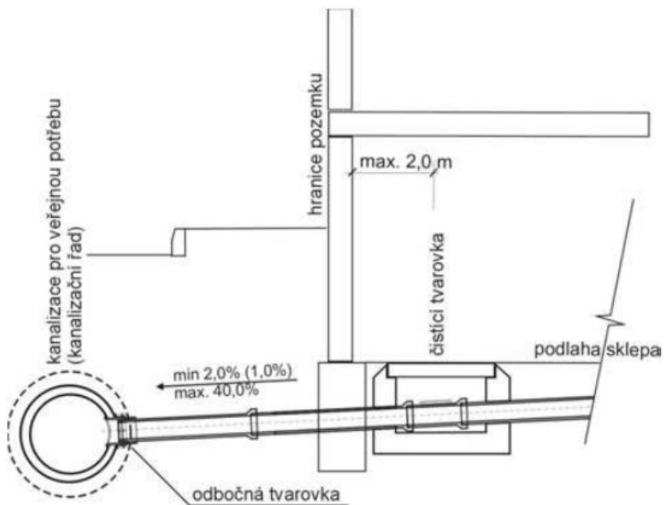
b) Schéma s čistící tvarovkou na kanalizační přípojce v půdorysu objektu v podlaze
